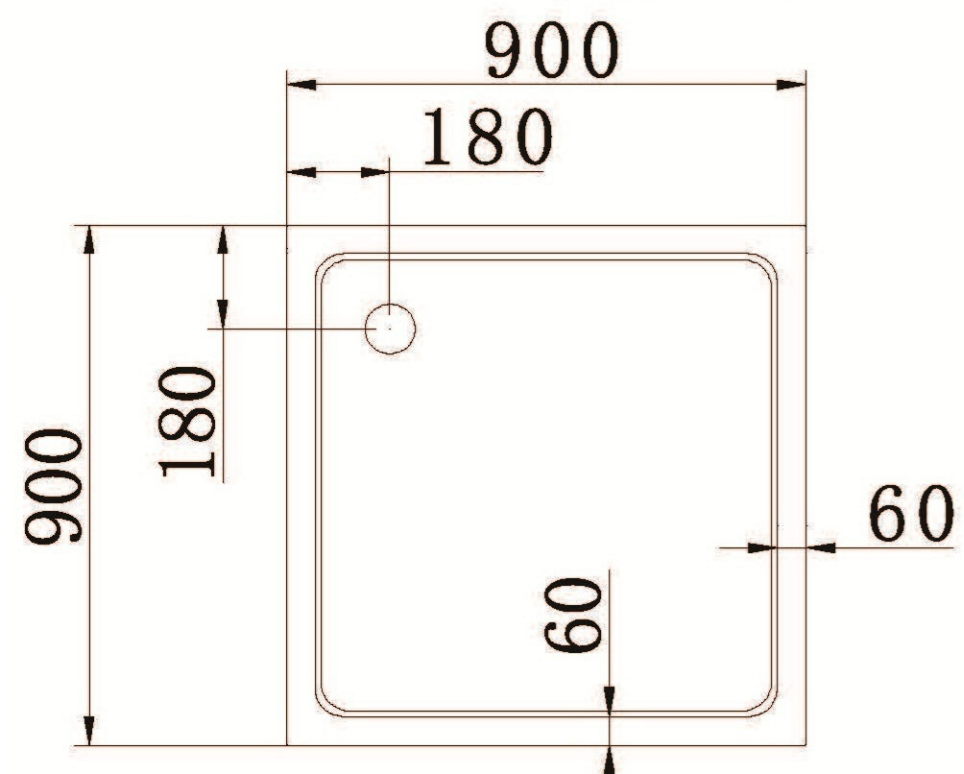
TRAY-A-A-90-15 .. (поддон акриловый)
